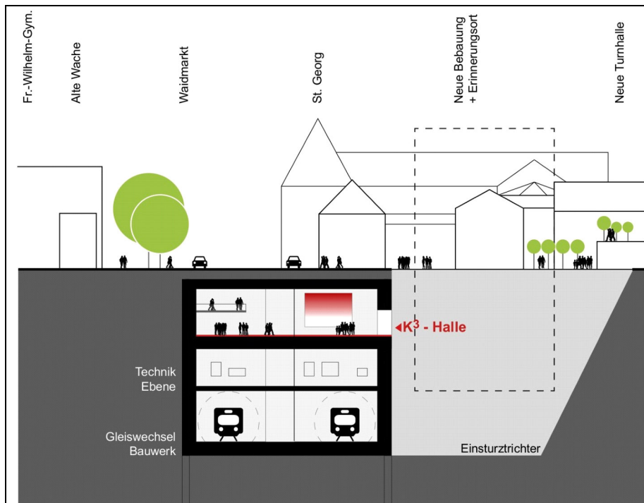
Querschnitt KVB-Bauwerk Severinstraße/Waidmarkt
